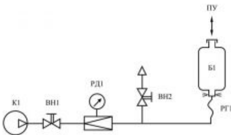
Схема установки для окраски вертикальных трубопроводов. K1 – компрессор (400 л/мин, 8 кг/см 2 ), BN1, BN2 – кран шаровый, Ду15, RD1 – регулятор давления с фильтром-влажностителем и манометром FR-200 (1500 л/мин, 1/4"), PG1 – гибкий рукав (Ду9, L = 80 м), B1 – бачок с форсункой, ПУ – подъемное устройство.
